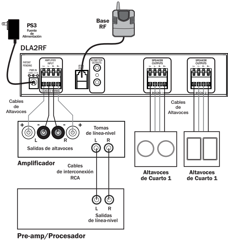
Dibujo 2-4: Aplicación de Amplificador - Procesador/Pre-amp
